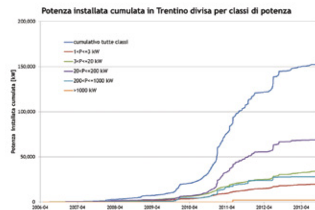
Figura 2: Potenza installata cumulata in Trentino divisa per classi di potenza.
