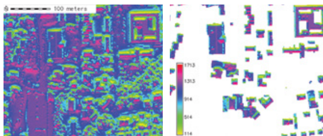
Figura 13: A sinistra, mappa della radiazione solare totale annua corretta con i dati misurati a terra. A destra, estrazione degli edifici dalla mappa della radiazione
