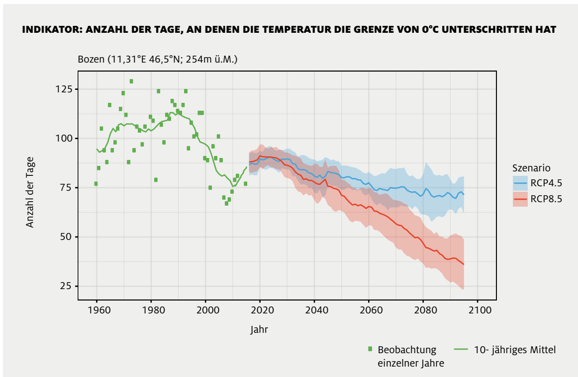
Abb. 39: Anzahl der Tage, an denen die Temperatur die Grenze von 0°C unterschritten hat. (Daten: WISKI Datenbank, Autonome Provinz Bozen. Darstellung: Eurac Research)
