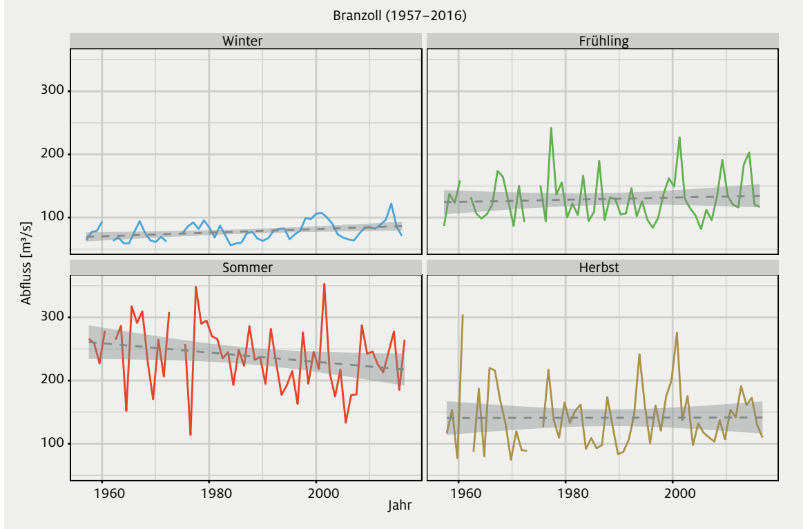
Abb. 19: Jahreszeitliche Trends bei den mittleren monatlichen Abflüssen der Etsch in Branzoll (Jahre 1957–2016). (Daten und Darstellung: Hydrographische Amt, Autonome Provinz Bozen)
