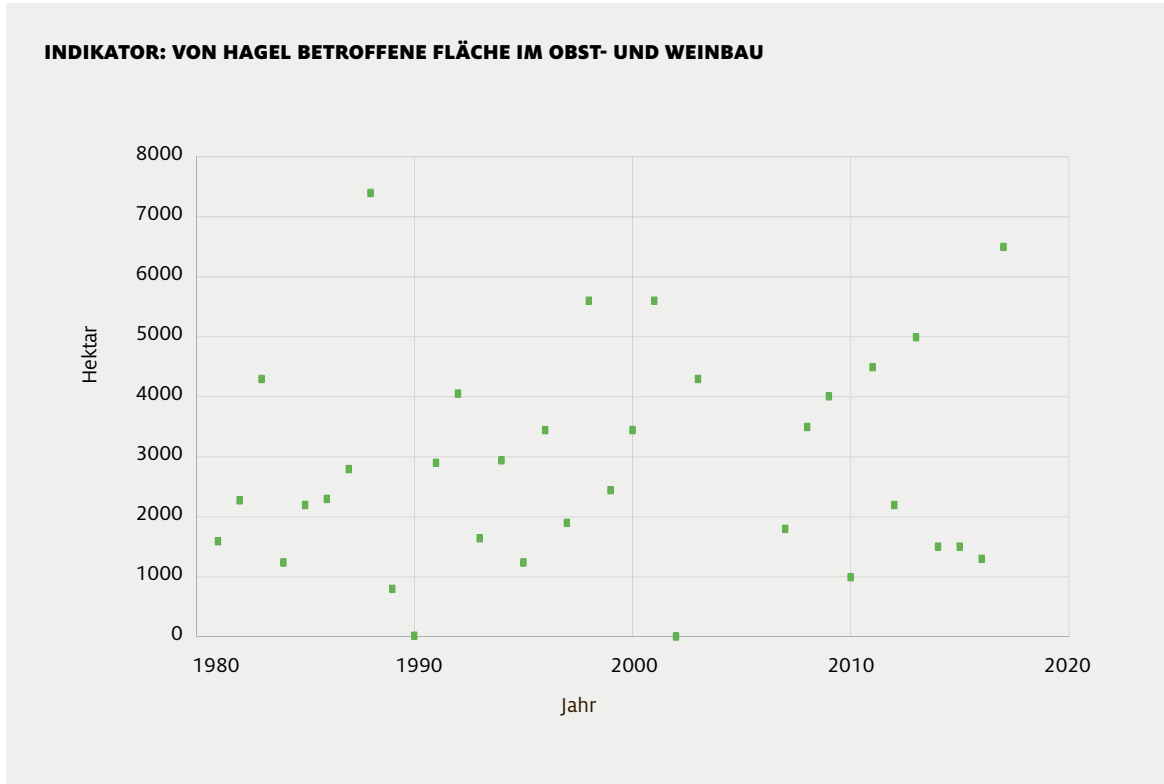
Abb. 30: Schätzungen der vom Hagel betroffenen Fläche im Obst- und Weinbau lassen statistisch keine signifikante Zunahme erkennen; die verfügbaren Daten sagen allerdings nichts über die Schwere der Schäden aus. (Daten: Hagelschutzkonsortium Südtirol. Darstellung: Eurac Research)
