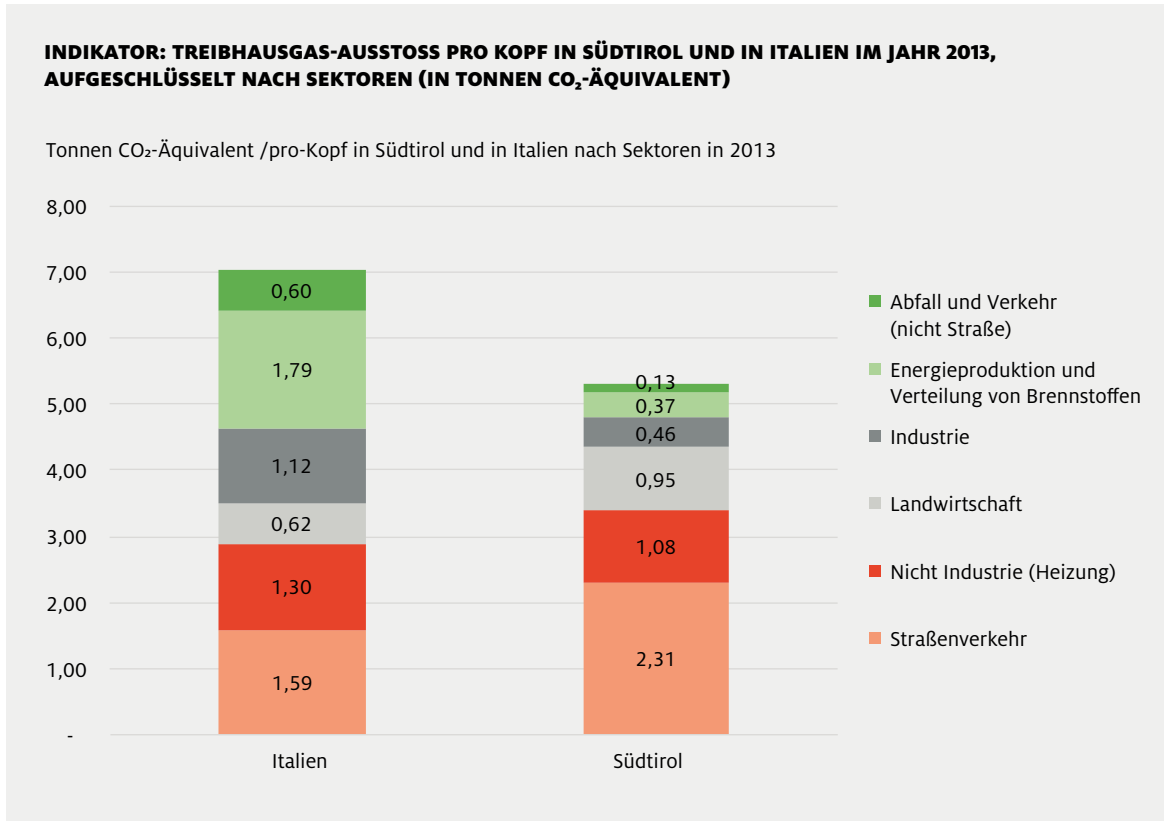
Abb. 12: t Tonnen CO 2 -Äquivalent /pro-Kopf in Südtirol und in Italien nach Sektoren in 2013. (Daten: ISPRA, Amt für Luft und Lärm, Autonome Provinz Bozen. Darstellung: Eurac Research)
