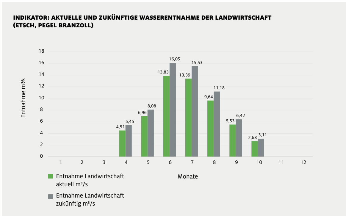
Abb. 28: Monatliche Wasserentnahmen für die Landwirtschaft in der Provinz Bozen, bezogen auf das Einzugsgebiet der Etsch. Angegeben werden die aktuellen Wasserentnahmen sowie die von der Provinzverwaltung für die nächsten 30 Jahre vorhergesehenen. (Daten: Gesamtplan für die Nutzung der öffentlichen Gewässer der Autonomen Provinz Bozen. Darstellung: Eurac Research)
