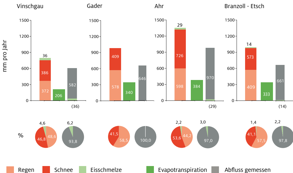
Abb. 17: Wasserbilanz der Etsch und einiger Nebenflüsse für die Jahre 1990 – 2010. Die Bilanz ist in Millimeter pro Jahr und als Prozentwert angegeben. Hervorgehoben sind die Zuflüsse durch Regen und durch die Schnee- und Gletscherschmelze, Verluste durch Evapotranspiration sowie die Abflüsse. (Daten und Darstellung: Hydrographische Amt, Autonome Provinz Bozen)
