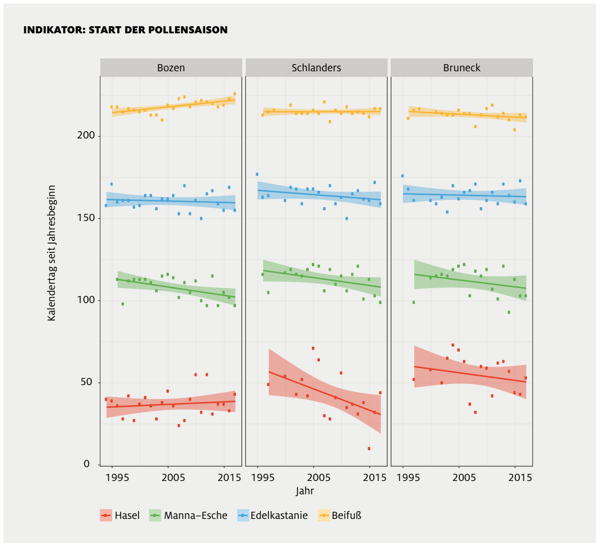
Abb. 24: Start der Pollensaison an drei Standorten in Südtirol von 1994-2017. (Daten: Landesumweltagentur, Autonome Provinz Bozen. Darstellung: Eurac Research)
