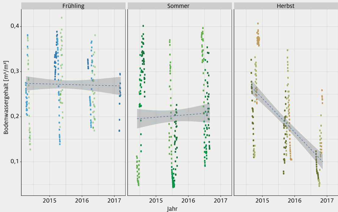
Abb. 25: Während im Frühling und im Sommer keine Veränderungen feststellbar sind, ist der Bodenwassergehalt im Herbst in den letzten drei Jahren geringer geworden. Für längerfristige Aussagen muss die Messreihe allerdings noch über mehrere Jahre fortgeführt werden. (Daten und Darstellung: Eurac Research)
