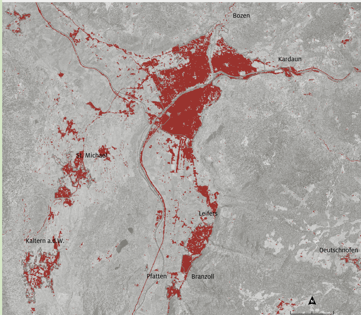
Abb. 34: Bodenversiegelung in der Gemeinde Bozen und Umgebung, 2012. Kartierung basiert auf hochauflösenden Satellitendaten. (Daten: Europäische Umweltbehörde EEA. Darstellung: Eurac Research)
