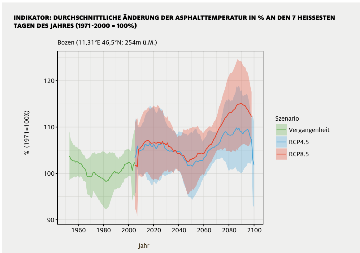
Abb. 40: Durchschnittliche Änderung der Asphalttemperatur in % an den 7 heißesten Tagen des Jahres (1971-2000 = 100 %). (Daten: WISKI Datenbank, Autonome Provinz Bozen. Darstellung: Eurac Research)
